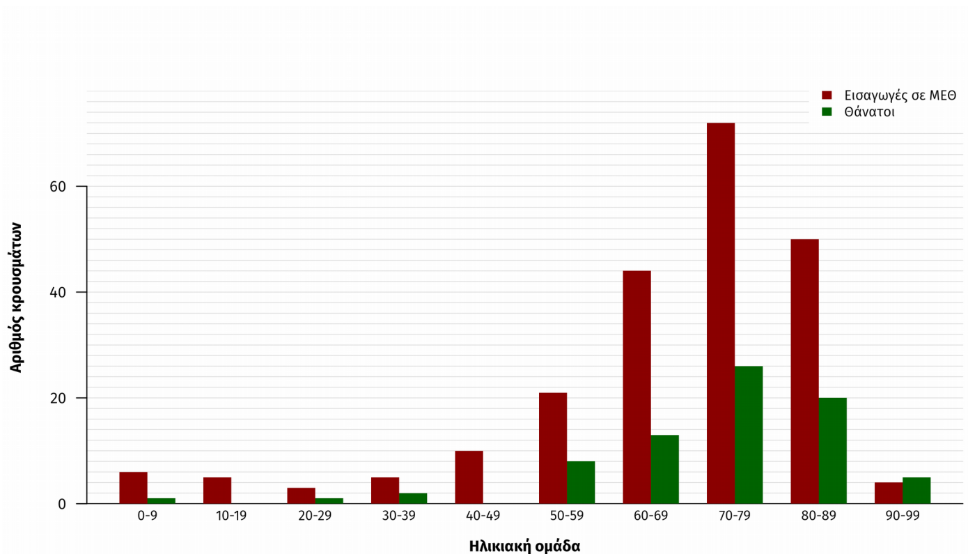
Διάγραμμα 6: Ηλικιακή κατανομή εισαχθέντων σε Μ.Ε.Θ. με εργαστηριακά επιβεβαιωμένη γρίπη και ασθενών που κατέληξαν σε Μ.Ε.Θ ή εκτός Μ.Ε.Θ. Σύνολο Ελλάδας, από εβδομάδα 40/2016 έως εβδομάδα 8/2017 (20-26 Φεβρουαρίου 2017).
