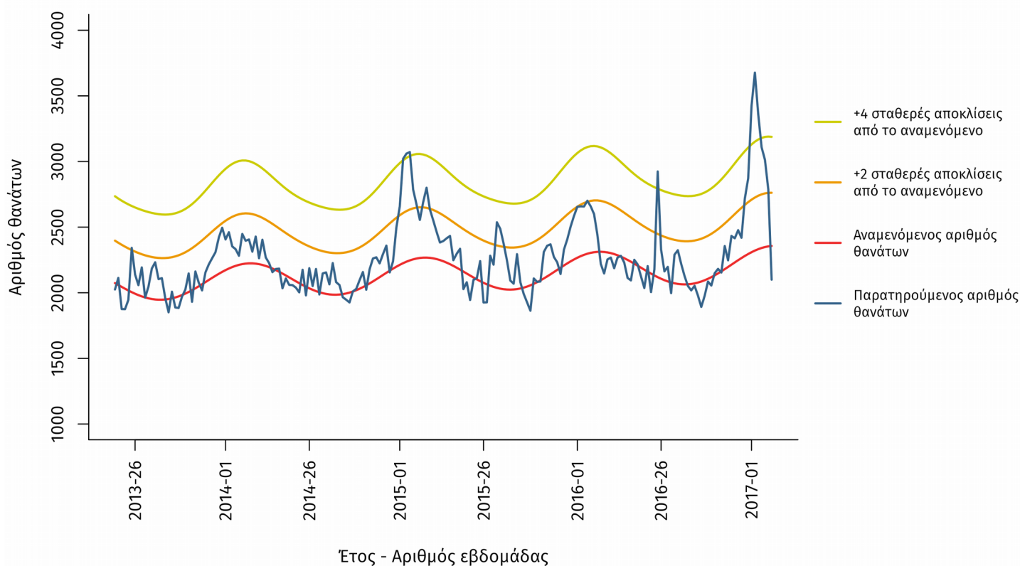
Διάγραμμα 7: Παρατηρούμενος και αναμενόμενος αριθμός θανάτων κατά εβδομάδα στις περιοχές της Ελλάδας που μετέχουν στο σύστημα επιτήρησης. Εβδομάδα 20/2013 έως εβδομάδα 8/2017.
