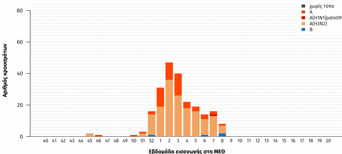
Διάγραμμα 4: Αριθμός εισαγωγών σε Μ.Ε.Θ. ανά εβδομάδα, σε ασθενείς με εργαστηριακά επιβεβαιωμένη γρίπη. Σύνολο Ελλάδας, από εβδομάδα 40/2016 έως εβδομάδα 8/2017 (20-26 Φεβρουαρίου 2017). Συνολικός αριθμός δηλωθέντων κρουσμάτων έως και την εβδομάδα 8/2017: 220
