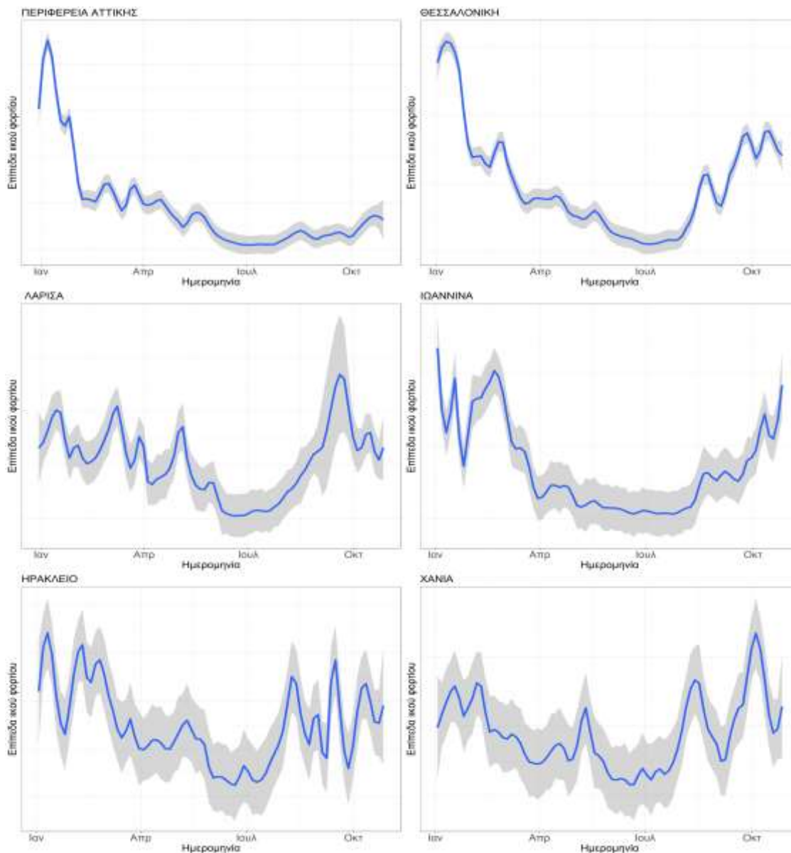
Διάγραμμα 19: Διακύμανση επιπέδων ιικού φορτίου (γονιδιωματικά αντίγραφα/100.000 πληθυσμό) στα αστικά λύματα συναρτήσει του χρόνου κατά την περίοδο 29/12/2022-29/10/2023
