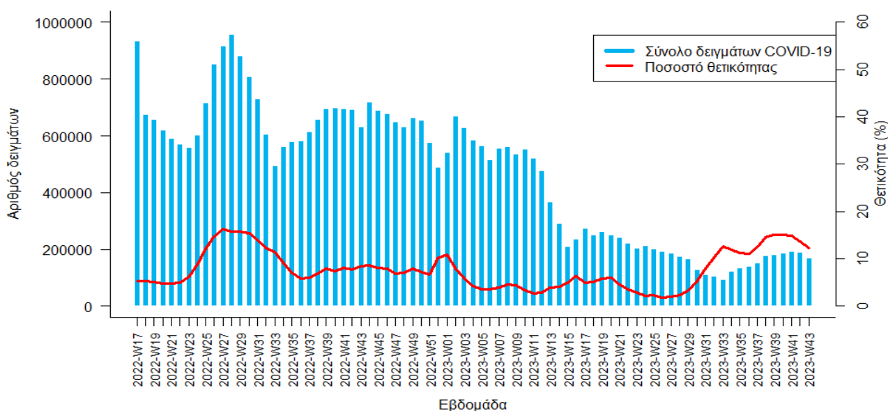
Διάγραμμα 7. Σύνολο δειγμάτων (Rapid-Ag/Rt-PCR) και ποσοστό θετικότητας με βάση το σύνολο των ελεγχθέντων δειγμάτων COVID-19, εβδομάδα 17/2022 - εβδομάδα 43/2023
