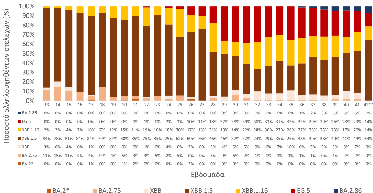
Διάγραμμα 17. Ποσοστό αλληλουξηθέντων δειγμάτων με απομονωθέν στέλεχος BA.2 ανά υπο-παραλλαγή επιδημιολογικού ενδιαφέροντος, ανά εβδομάδα, έως 18/10/2023
