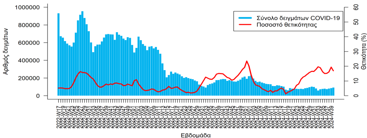
Διάγραμμα 7. Σύνολο δειγμάτων (Rapid-Ag/Rt-PCR) και ποσοστό θετικότητας με βάση το σύνολο των ελεγχθέντων δειγμάτων COVID-19, εβδομάδα 17/2022 - εβδομάδα 40/2024
