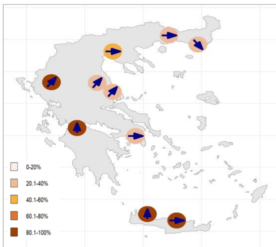
Εικόνα 2: Γεωγραφική απεικόνιση των επιπέδων ιικού φορτίου στα αστικά λύματα και τάση μεταβολής κατά την εβδομάδα 40/2024
