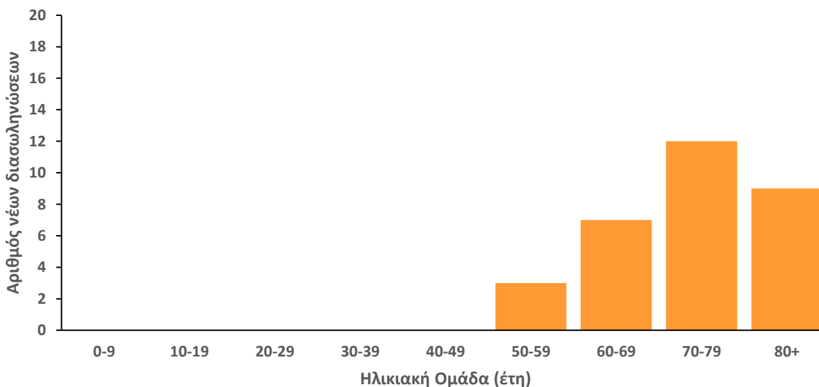
Διάγραμμα 10. Αριθμός νέων διασωληνώσεων ασθενών με λοίμωξη COVID-19 στα νοσοκομεία της επικράτειας ανά ηλικιακή ομάδα, εβδομάδα 37/2024 – εβδομάδα 40/2024
