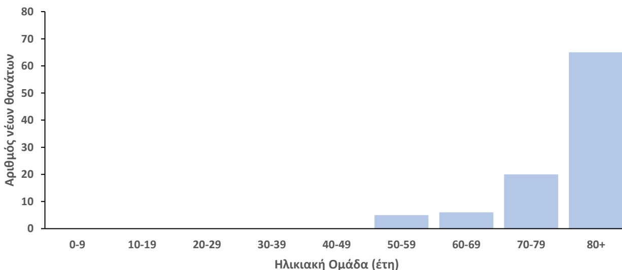
Διάγραμμα 14. Αριθμός θανάτων COVID-19 ανά ηλικιακή ομάδα, εβδομάδα 37/2024 – εβδομάδα 40/2024
