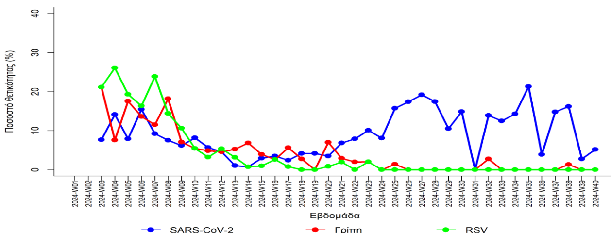
Διάγραμμα 6. Ποσοστό θετικότητας ρινοφαρυγγικών δειγμάτων για SARS-CoV-2, ιούς γρίπης και αναπνευστικό συγκυτιακό ιό (RSV), από ασθενείς με Σοβαρή Οξεία Λοίμωξη Αναπνευστικού (SARI), Δίκτυο Επιτήρησης SARI, σύνολο χώρας, εβδομάδα 03*/2024 – εβδομάδα 40/2024
