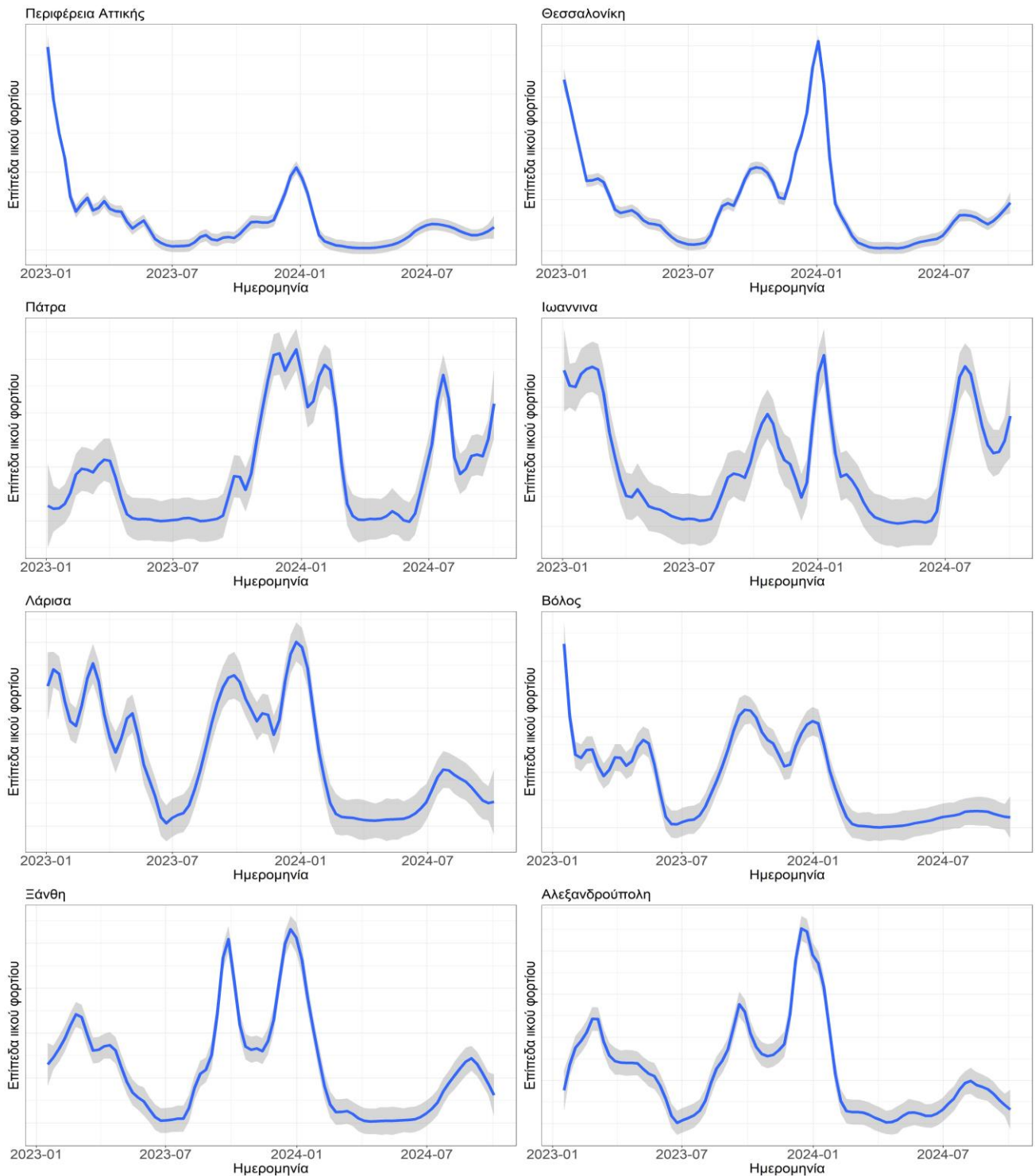
Διάγραμμα 16: Διακύμανση επιπέδων ιικού φορτίου (γονιδιαστικά αντίγραφα/100.000 πληθυσμό) στα αστικά λύματα συναρτήσει του χρόνου κατά την περίοδο 01/01/2023-06/10/2024
