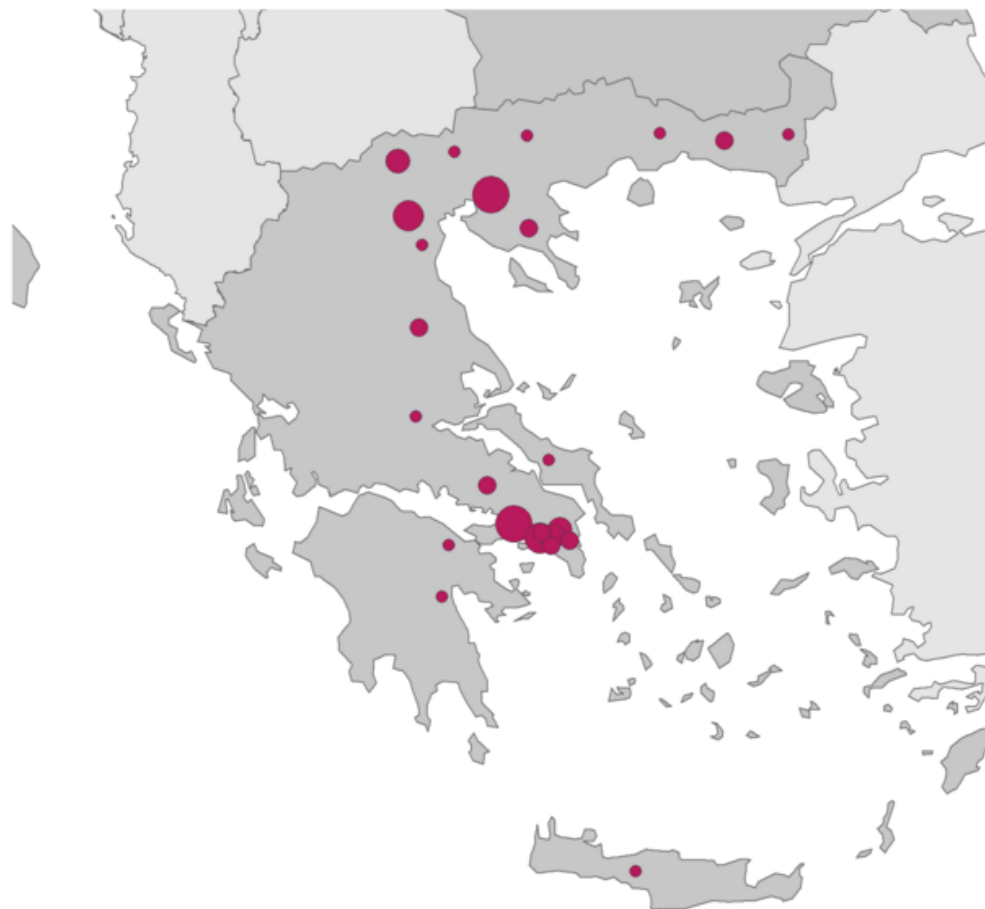
Εικόνα 2: Διαβάθμιση αριθμού κρουσμάτων λοίμωξης από τον ιό του Δυτικού Νείλου (ΙΔΝ) ανά πιθανή Περιφερειακή Ενότητα έκθεσης, Ελλάδα, 2018 (n=312)*.
